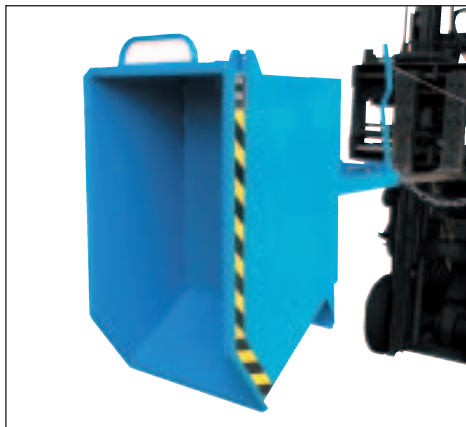
Typ SGU in Kippstellung
