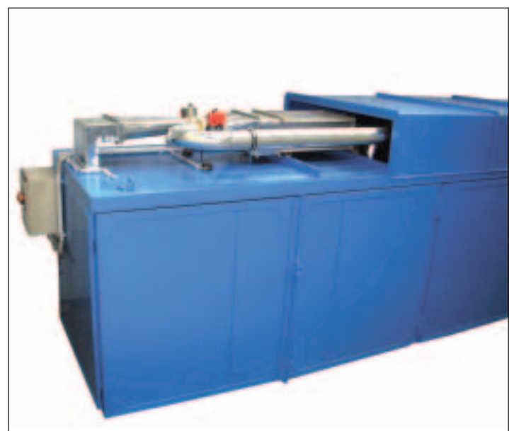
Typ WK mit Witterungsschutz der Heizungsrohre
